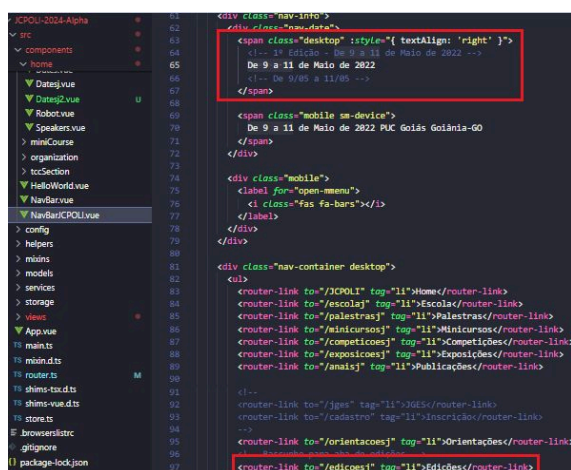
Figura 14 – Adição da data e aba “Edições” ao código da Escola Politécnica e de Artes.
