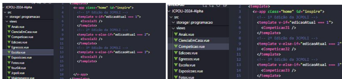
Figura 25 – Código dos arquivos “Escola.vue” e “Competicao.vue” com as chamadas de componentes.
