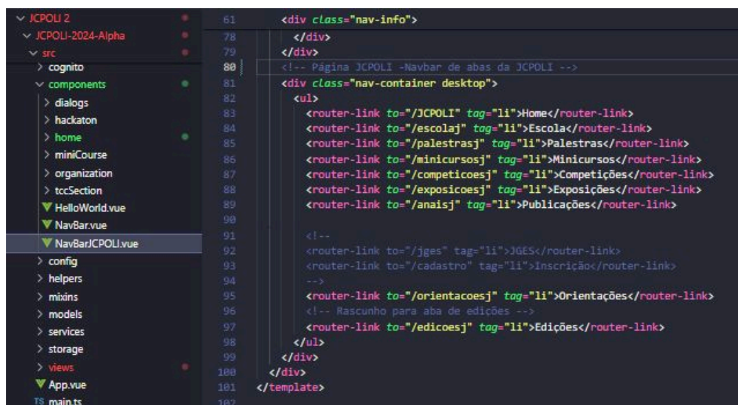
Figura 6 –Código da Politécnica com uma “NavBar” exclusiva para as abas da JCPOLI.
