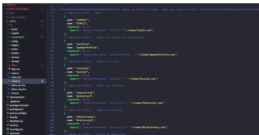
Figura 4 – Código da Escola Politécnica, na parte “router.ts” com rotas da JCPOLI.
